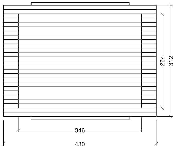
dessus 1:5
