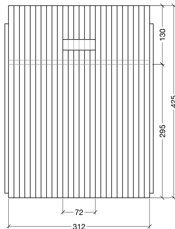
profil 1:5
