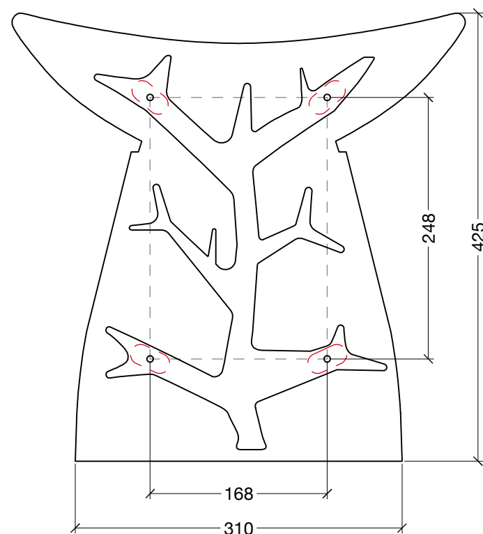
face 1:5
