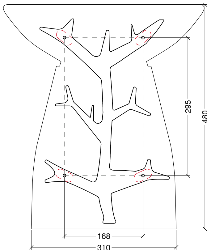
face 1:5
