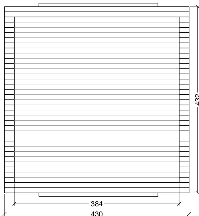
face 1:5
