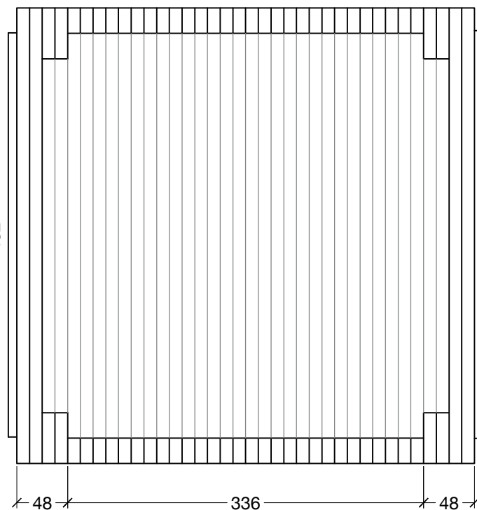
profil 1:5
