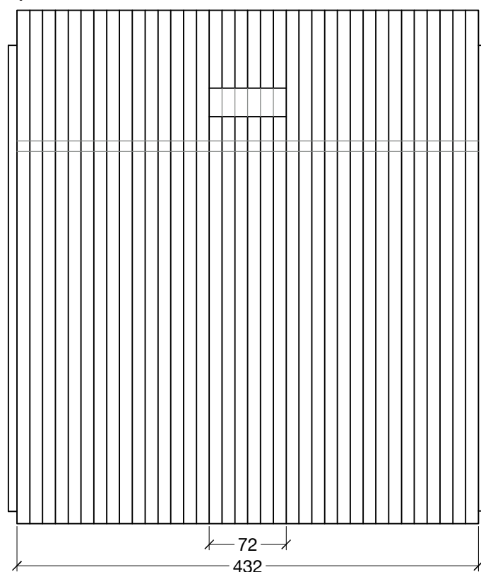
profil 1:5
